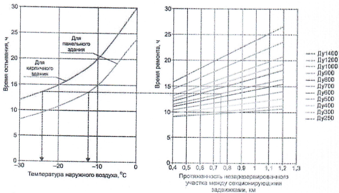
Рисунок 12 - Номограмма для определения периодов остывания для подъездов и лестничных клеток жилых зданий со снижением температуры с +15 до +3^{\circ}\text{C}
