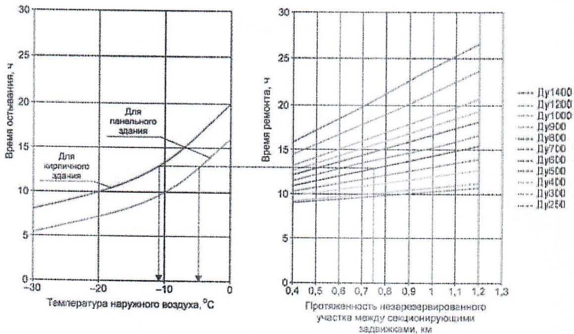
Рисунок 11 - Номограмма для определения периодов остывания угловых жилых помещений кирпичных и панельных зданий со снижением температуры внутреннего воздуха помещений с +20 до +12^{\circ}\text{C}
